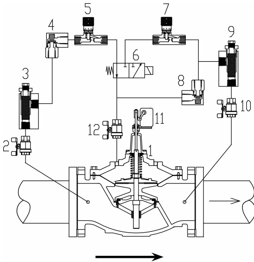
FIG. 2 Schematic A-0306C
