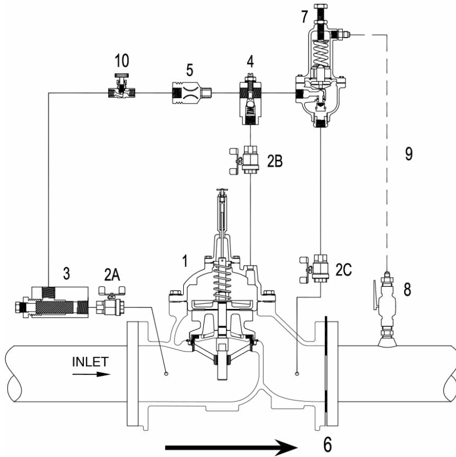
FIG. 2 Schematic A-7427C
